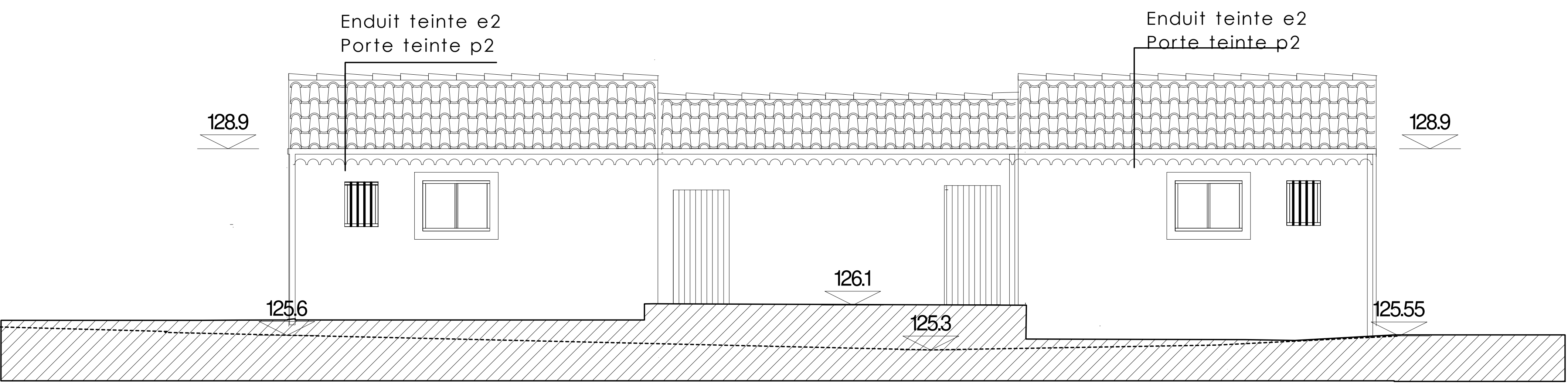
FACADES NORD VILLAS 17 ET 18
