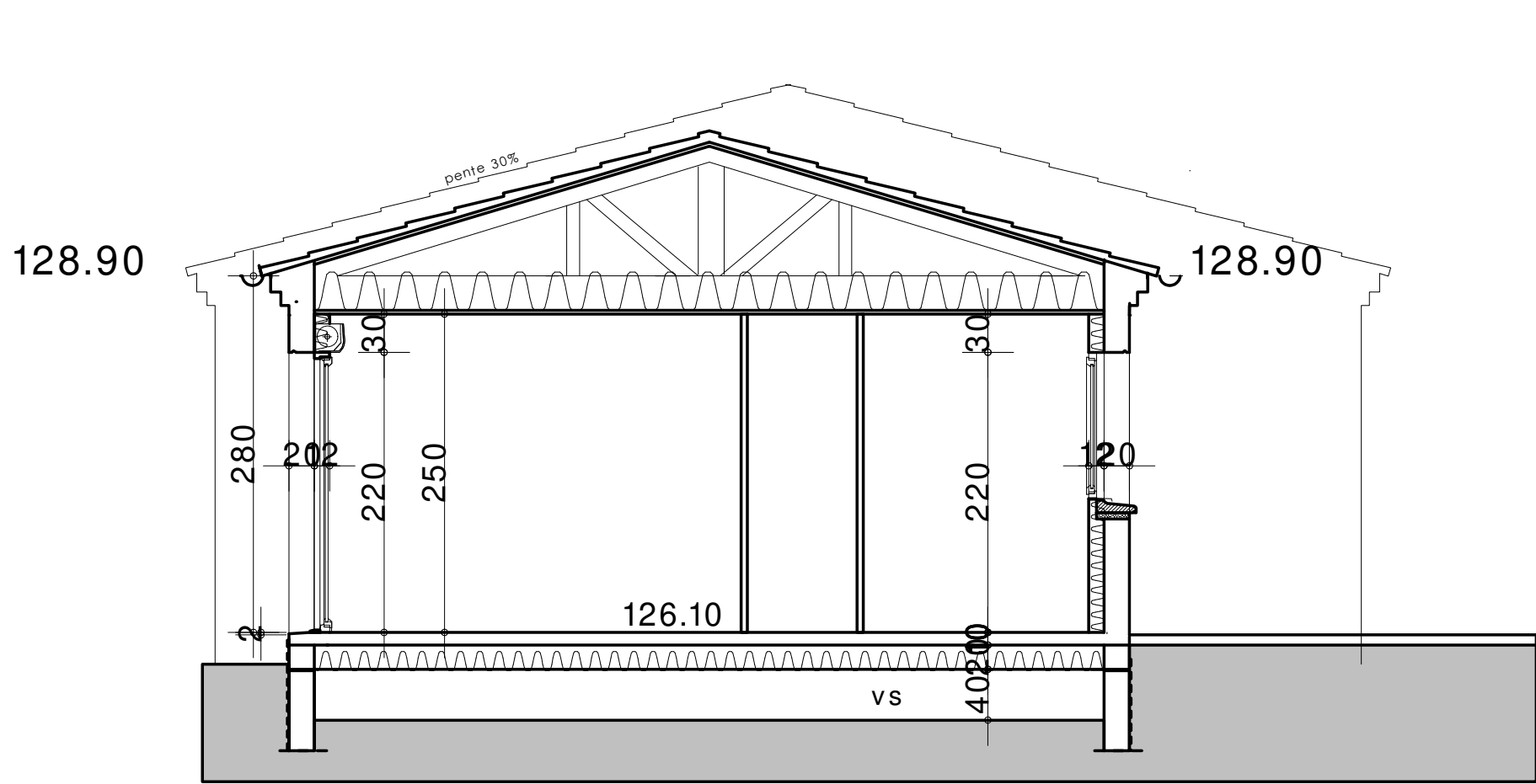
COUPE C-C
