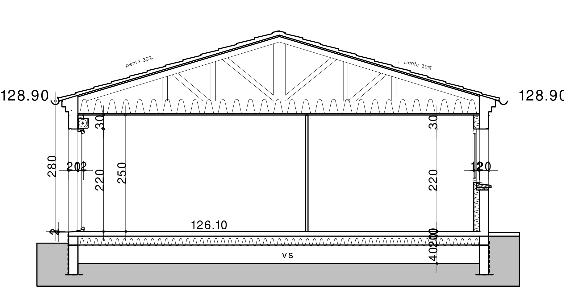
COUPE B-B
